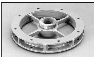
Estabilizador de Tipo Araña utilizado en un Super Screw
