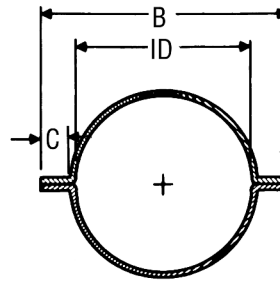
Artesa Tubular Bipartida con Ceja
