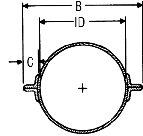
Artesa Tubular Bipartida con Ceja de Ángulo
