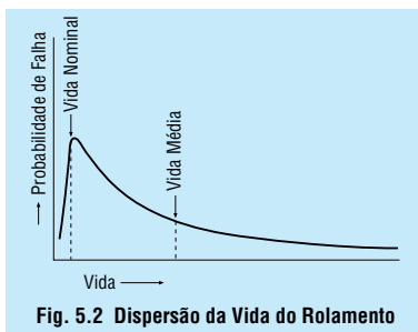
Fig. 5.2 Dispersão da Vida do Rolamento
