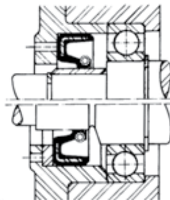
Recomendações de montagem
