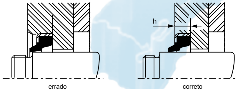
Detalhes de montagem
