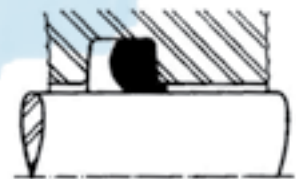
Vedação com extrusão
