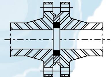
Vedação de flanges
