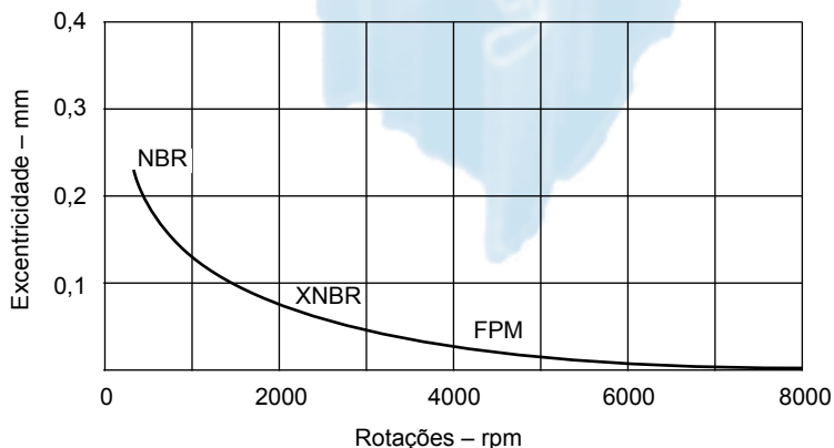
Excentricidade admissível aos eixos
