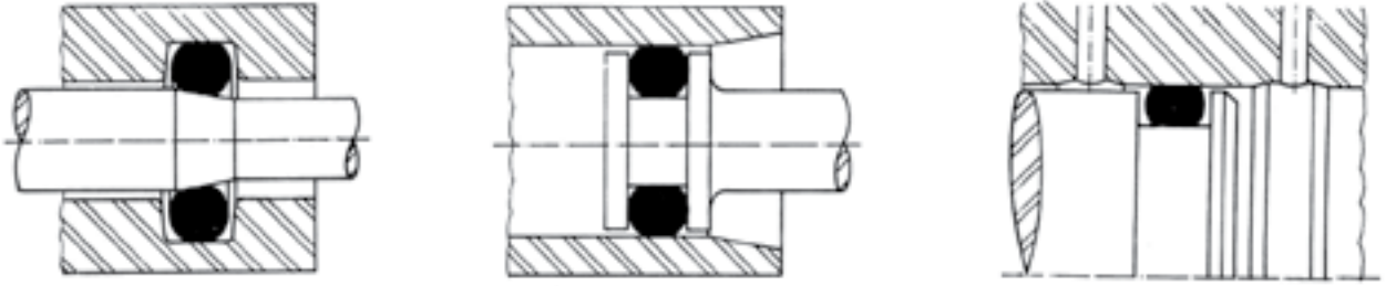
Detalhes de usinagem a serem observados
