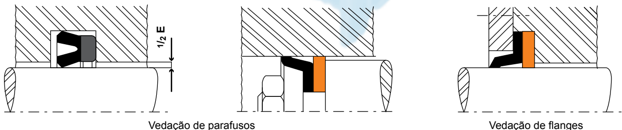
Vedação de parafusos
