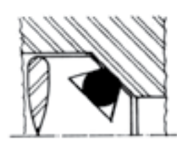
Assento de válvula
