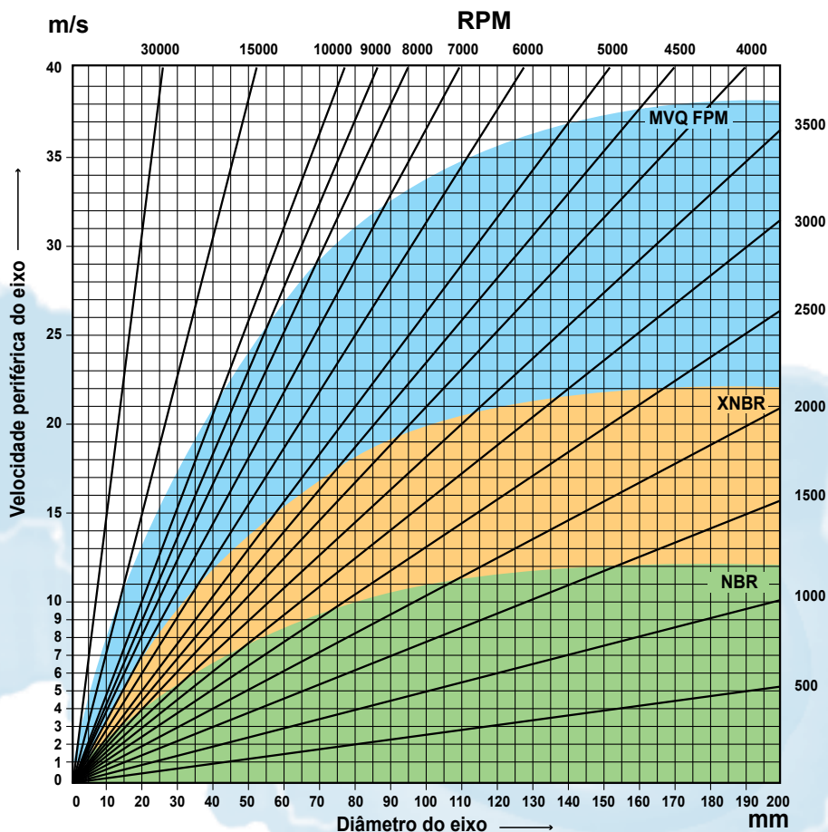
Velocidade periférica admissível aos retentores
