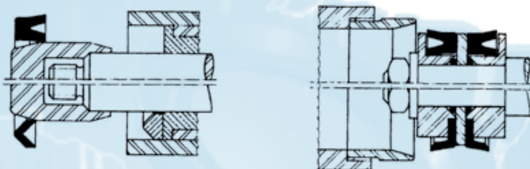
Dispositivos de montagem
