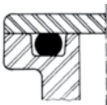
Deformação axial
