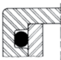
Deformação radial
